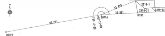
基準点網図 S-1/1000
